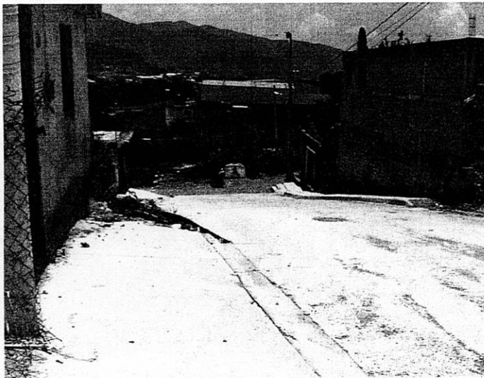
Pavimentación de Concreto Hidráulico en ingreso y calle La Providencia, Colonia Providencia. $1'247, 652.18
